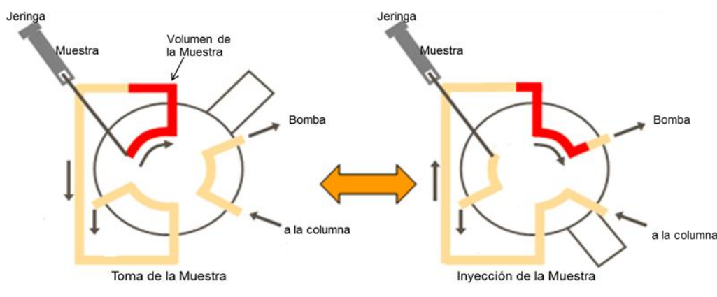
Figura 6. Válvula de inyección
