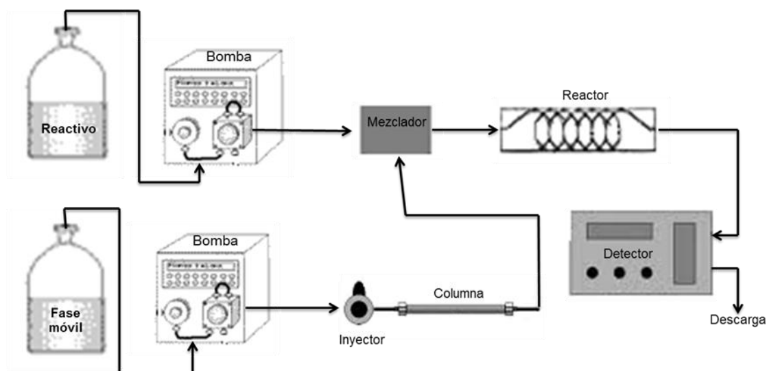
Figura 12. Esquema de un equipo de HPLC para operar con derivatización post columna
