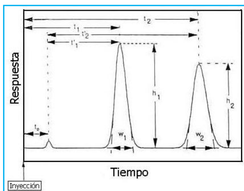
Figura 2. Cromatograma tipo
