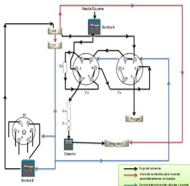
Figura 11. Esquema de un intercambio de columna para clean-up de muestras
