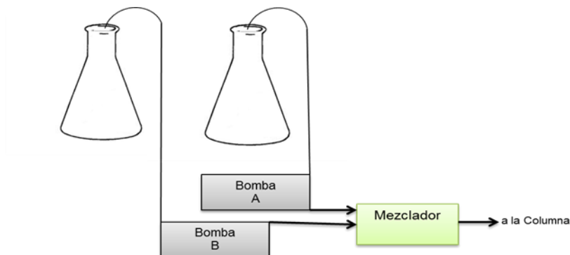
Figura 8. Sistema de formación de gradiente de alta presión
