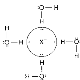
Anión hidratado
