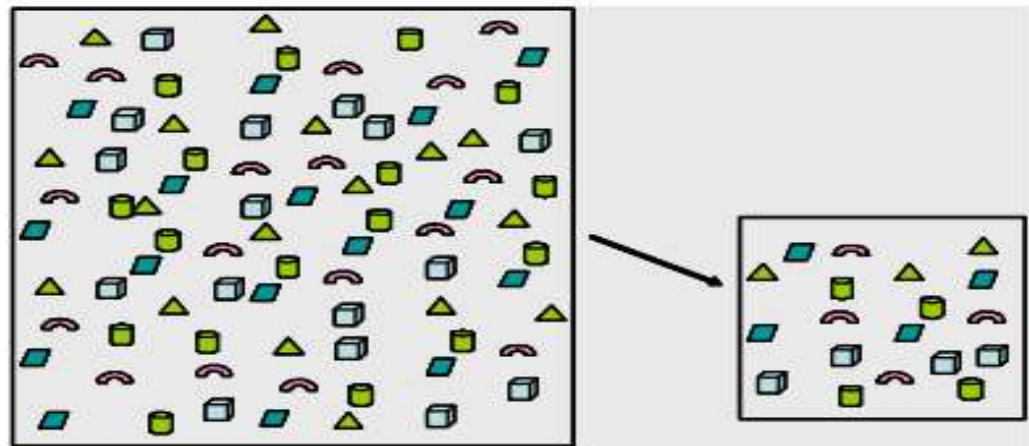
Figura 1. Representación gráfica del muestreo aleatorio simple.
